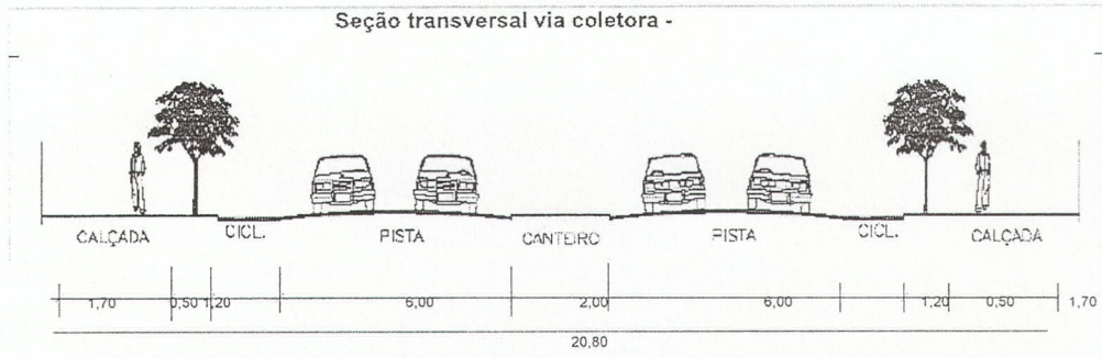
Seção transversal via coletora - desejável
